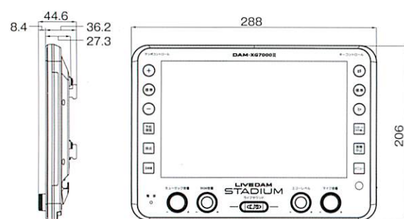
フロントパネル
